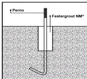
Fig 4. Anclar pernos
